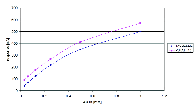
Figura 6. Curvas de calibración del potenciostato desarrollado (PSTAT110) y del potenciostato comercial TACUSSEIL RG.
