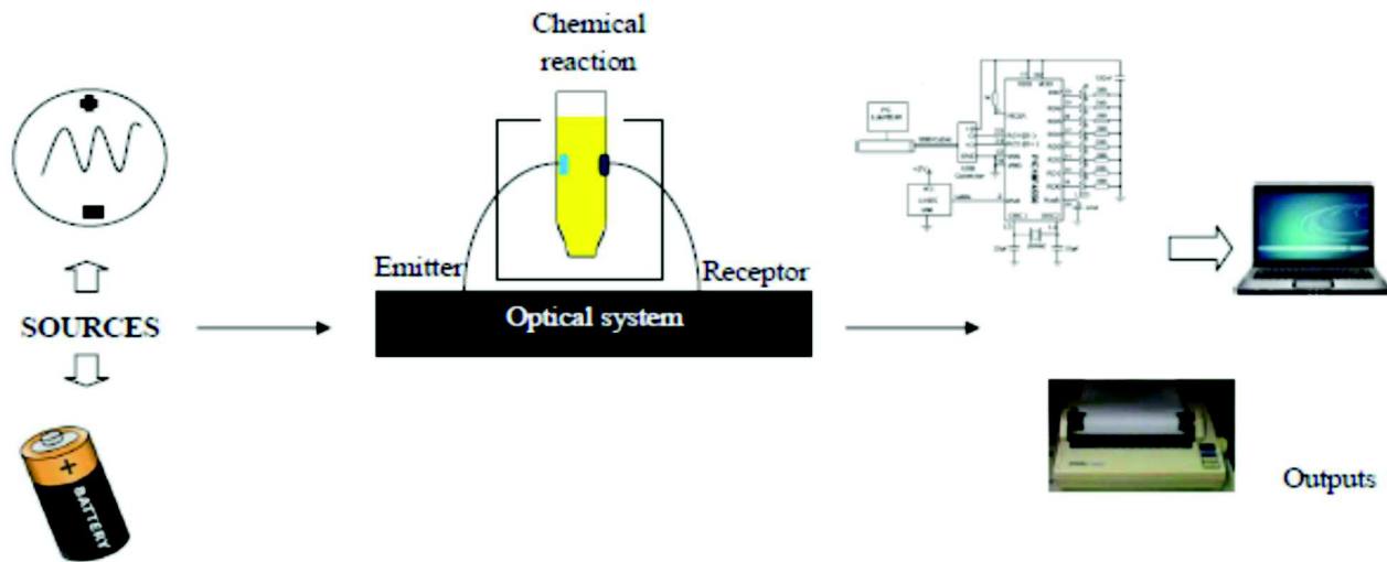
Figura 4. Esquema del espectrofotómetro desarrollado
