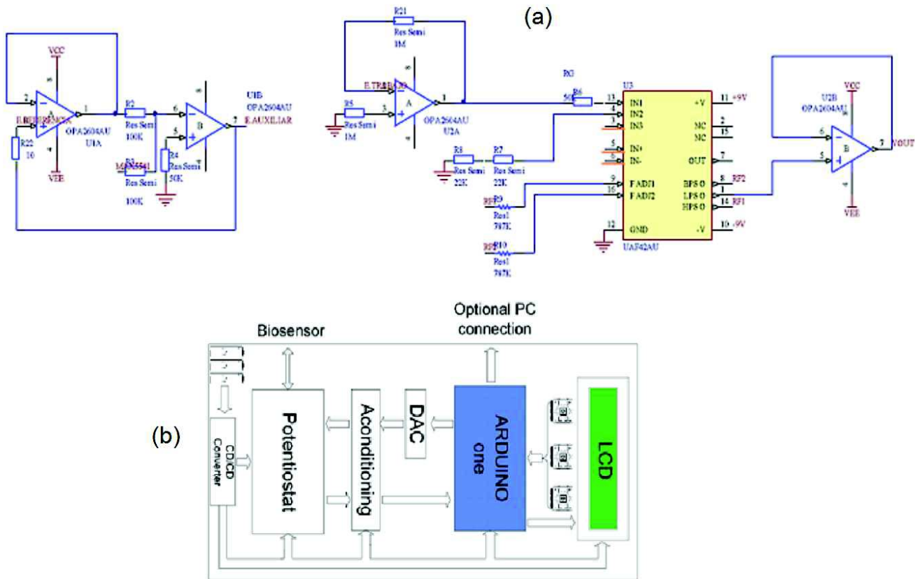
Figura 1. a). Esquema eléctrico del potenciostato desarrollado. b) El sistema del potenciostato completo, contiene algunos elementos que aseguran su portabilidad como lo son las baterías recargables la pantalla LCD todo controlado por una tarjeta Arduino Uno®.
