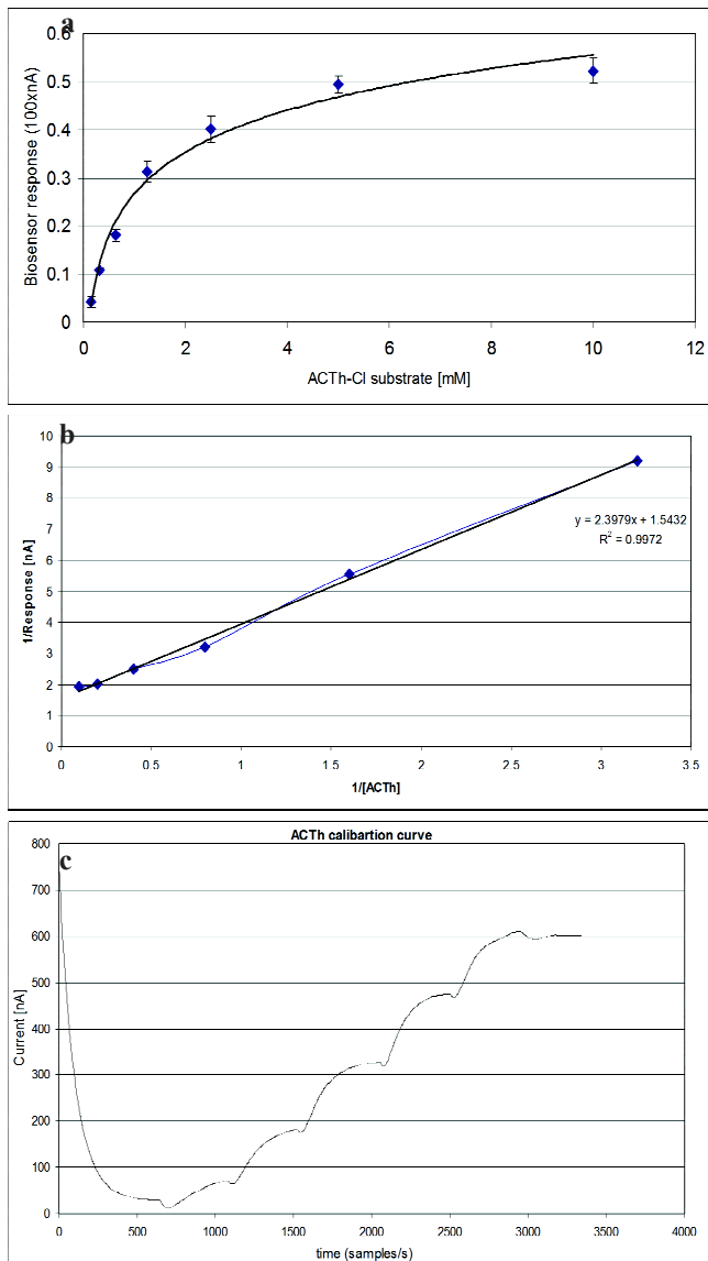
Figura 5. Detección del sustrato usando el potenciostato PSTAT110. a) Curva de correlación de la respuesta del potenciostato y de las concentraciones conocidas de ACTh-Cl. b) Curva doble inversa usada para calcular las constantes cinéticas de la enzima. c) inyecciones sucesivas de concentraciones cada vez más altas de ACTh-Cl.
