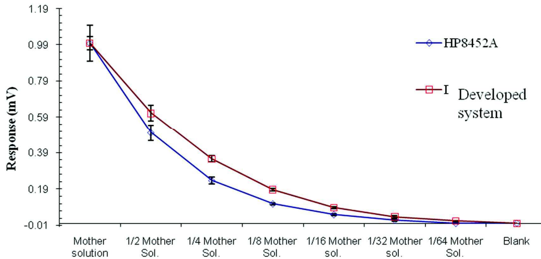
Figura 7. Curvas de calibración para nuestro espectrofotómetro y para el HP8452A.
