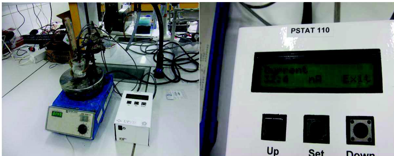
Figura 2. Potenciostato desarrollado
